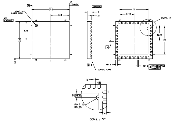
Si4684-A10-GM (QFN)
