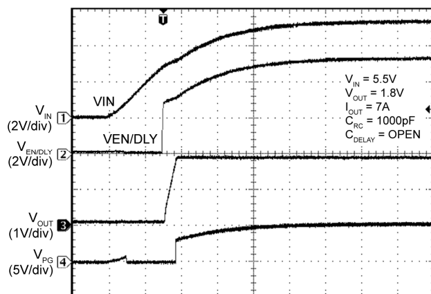
V_{IN} Turn-On
