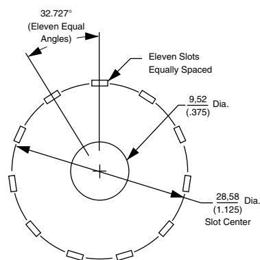
11R Socket
