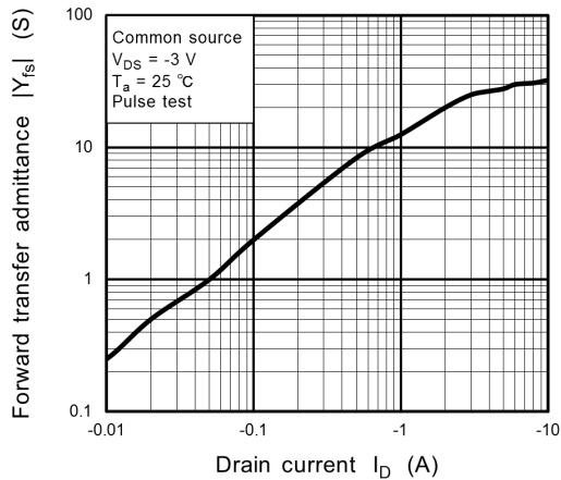
Fig. 7.7 |Y_{fs}| - I_D
