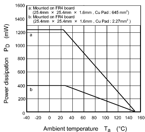
Fig. 7.13 P_D - T_a
