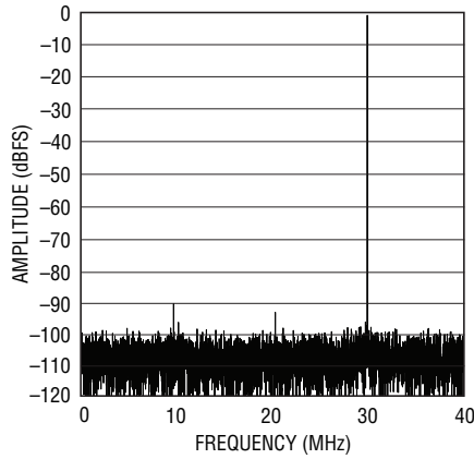
LTC2173-12: 8k Point FFT, f_{IN} = 30\text{MHz} -1\text{dBFS} , 80\text{Msps}
