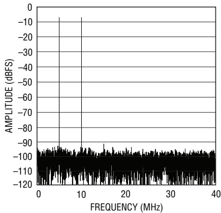
LTC2173-12: 8k Point 2-Tone FFT, f_{IN} = 70\text{MHz} , 75\text{MHz} , -1\text{dBFS} , 80\text{Msps}
