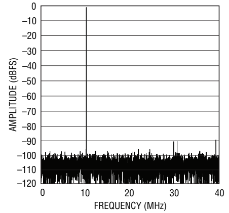
LTC2173-12: 8k Point FFT, f_{IN} = 70\text{MHz} -1\text{dBFS} , 80\text{Msps}
