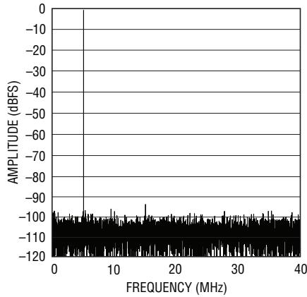
LTC2173-12: 8k Point FFT, f_{IN} = 5\text{MHz} -1\text{dBFS} , 80\text{Msps}
