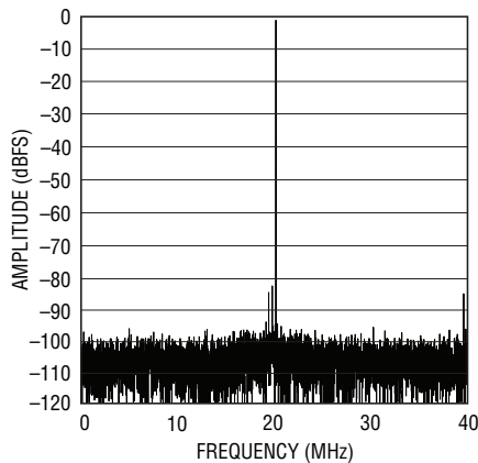
LTC2173-12: 8k Point FFT, f_{IN} = 140\text{MHz} -1\text{dBFS} , 80\text{Msps}
