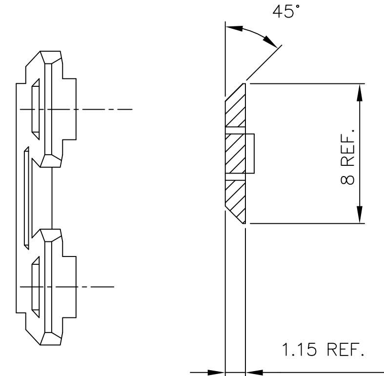
Section A-A
