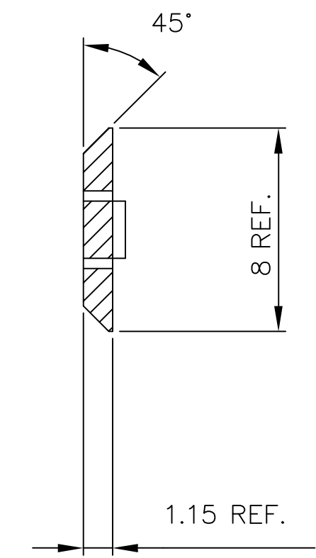
Section A-A
