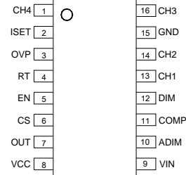
SO-16
