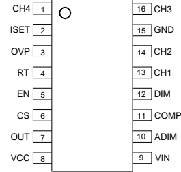
SO-16
