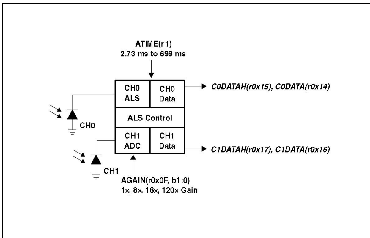
Figure 23: ALS Operation
