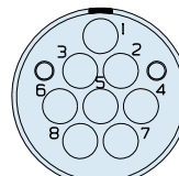
Size 15-08
