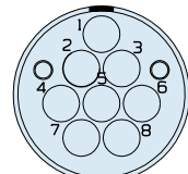
Size 15-08
