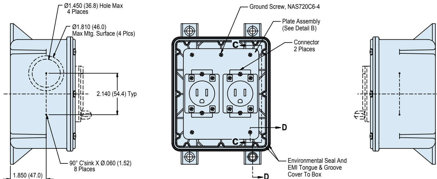
VIEW A-A
