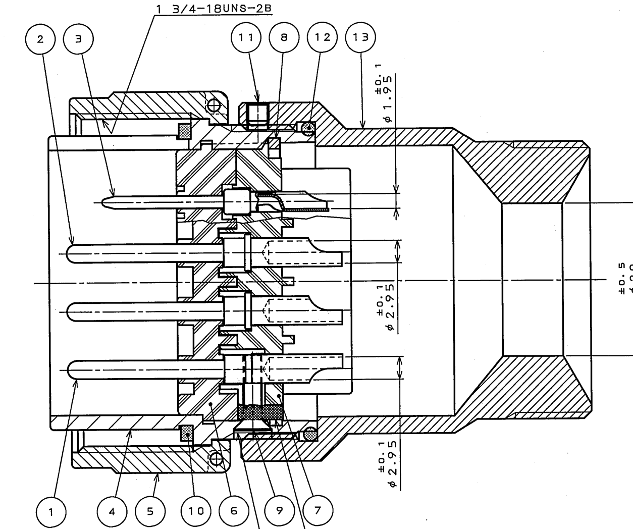
SECT-A-A (SCALE 2:1)
