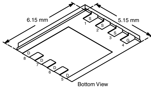
PowerPAK® SO-8
