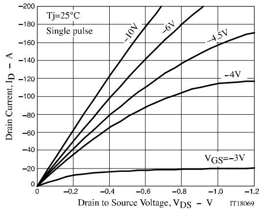
Figure 1. I_D - V_{DS}
