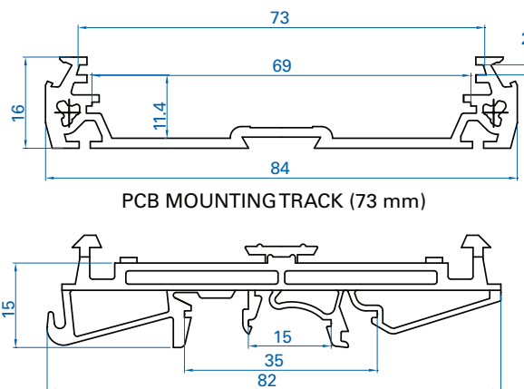
DIN RAIL MOUNTING FOOT (73mm)
