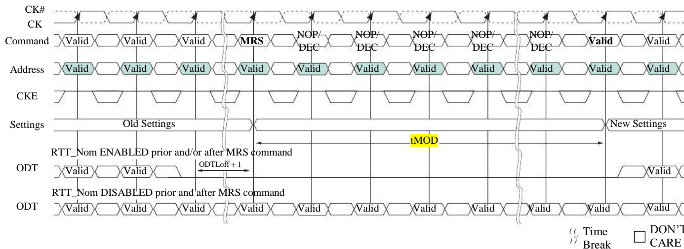
Figure 2.3.1b tMOD Timing
