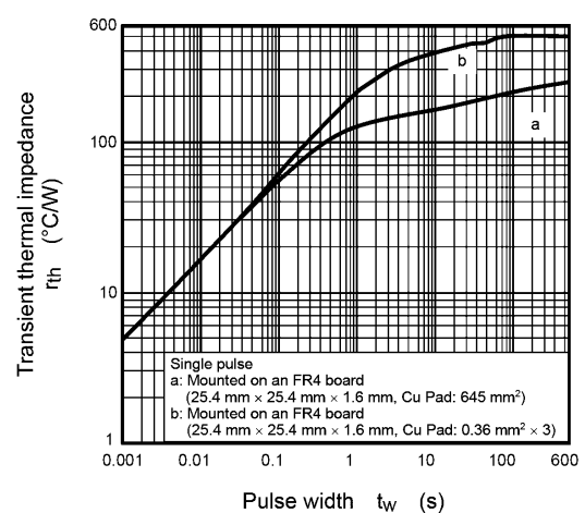
Fig. 7.12 r_{th} - t_w
