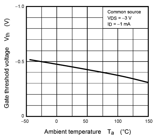
Fig. 7.6 V_{th} - T_a
