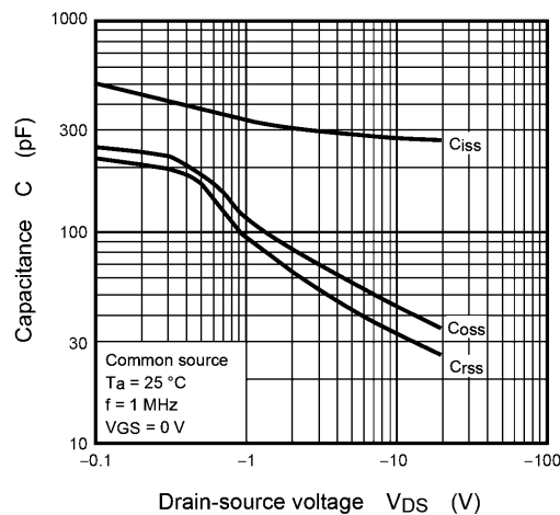
Fig. 7.9 C - V_{DS}
