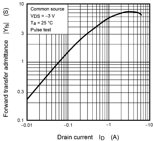
Fig. 7.7 |Y_{fs}| - I_D
