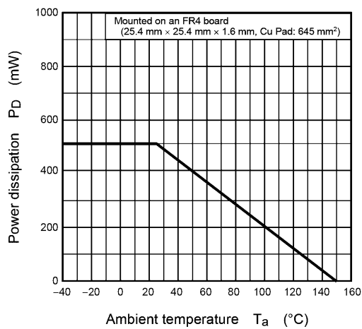
Fig. 7.13 P_D - T_a
