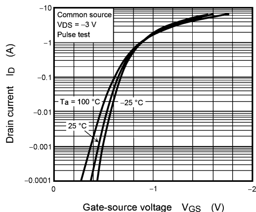
Fig. 7.2 I_D - V_{GS}
