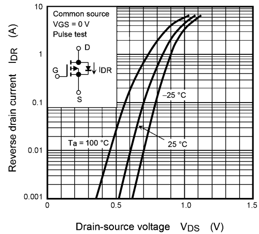
Fig. 7.8 I_{DR} - V_{DS}
