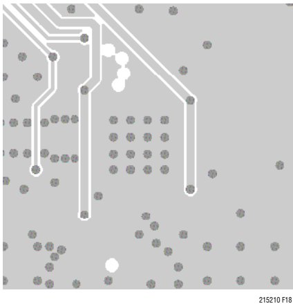
Inner Layer 4
