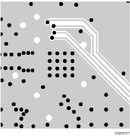
Inner Layer 3
