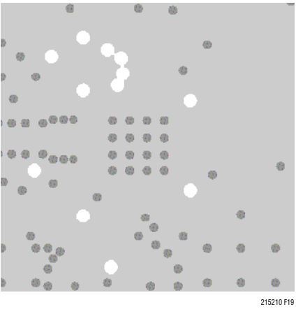
Inner Layer 5
