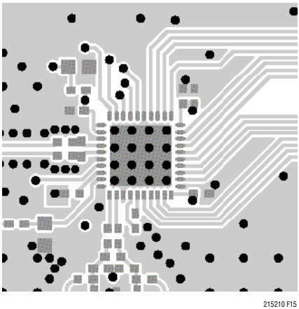
Inner Layer 1
