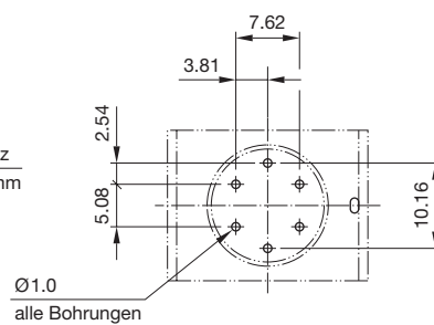
Bohrplan (Lötseite)
